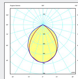
Curva de distribución luminosa
