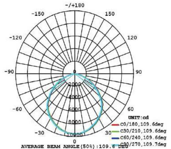
Curva de Distribución Luminosa
